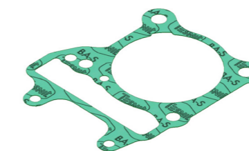
P02E000004858 12191-KZR-600 CYLINDER BASE GASKET / JUNTA CILINDRO (0,30 MM)
