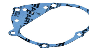
P003000004572 1B9-15461-00 TRANSMISSION COVER GASKET / JUNTA TAPA TRANSMISIÓN
